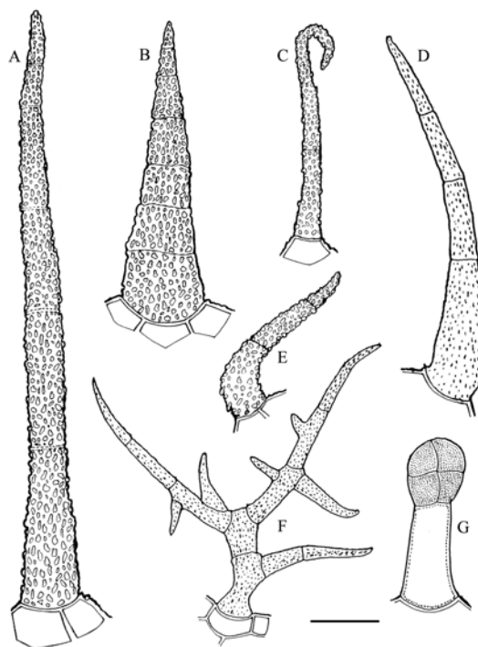
Fig. 1. Tipos de tricomas en Capsicum . A-B: Eglandular simple recto (Tipo I). C-E: Eglandular simple curvo (Tipo I). F: Eglandular ramificado (Tipo II). G: Glandular simple (Tipo III). Escalas: A-F: 100 \mu\text{m} , G: 50 \mu\text{m} .
